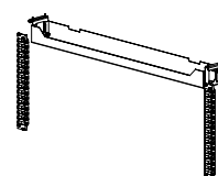
absenkbare Kabelwanne hinged cable tray
