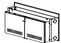
Türen vorne, abnehmbare Rückwand front doors, removable back panel
